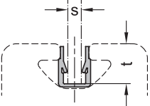
边缘型材
