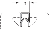
使用 盖型材
